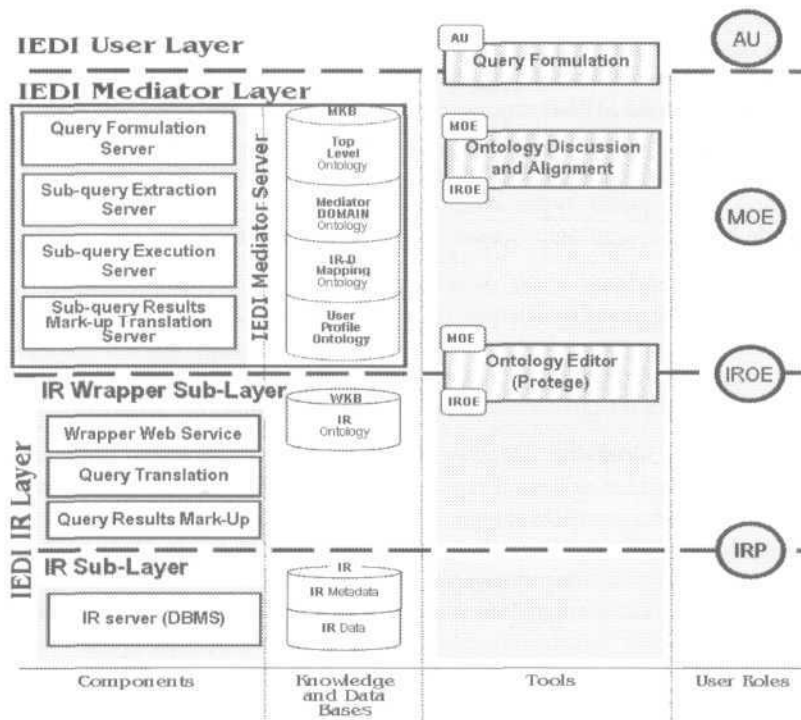
Figure 2. Clients et serveurs d'IIDE le long des couches de l'architecture.
