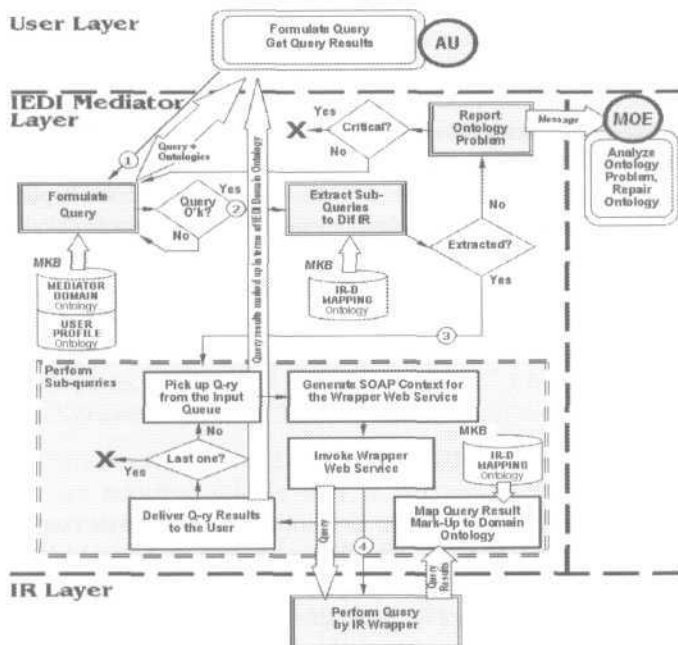
Figure. 1. Diagramme de processus pour le scénario d'exécution de demande d'IIDE.
